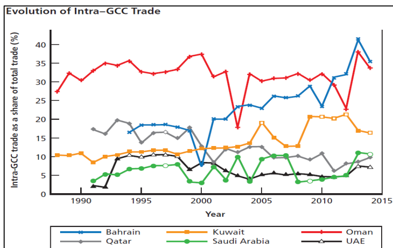
نمودار ۱. حجم تجارت درون منطقه‌ای کشورهای عضو شورای همکاری خلیج فارس (درصد از کل تجارت) (Rand Corporation, ۲۰۱۶, p. ۲۱)
